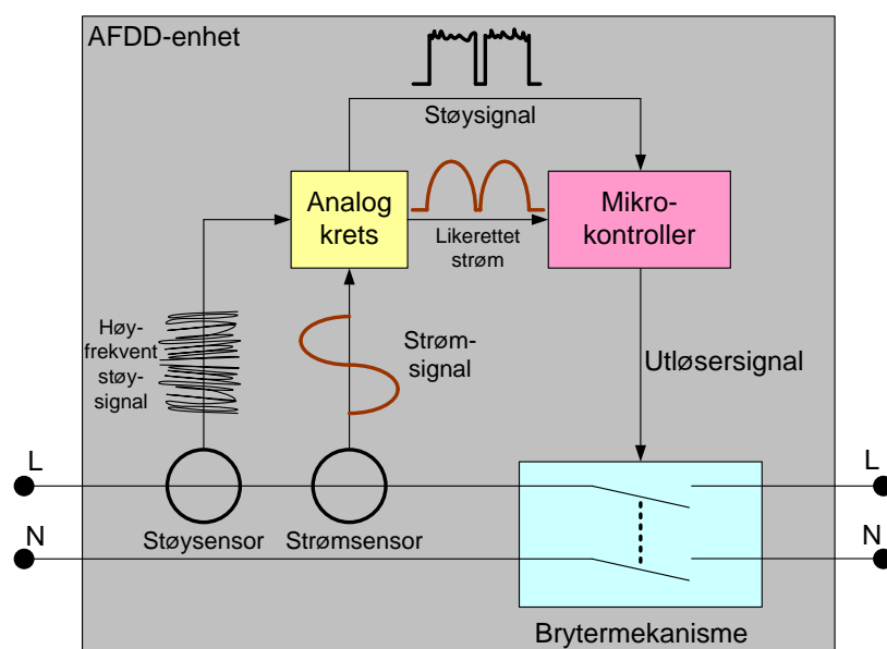
Figur 4: Prinsippskisse for designet til et Siemens 5SM6 lysbuevern [34].
